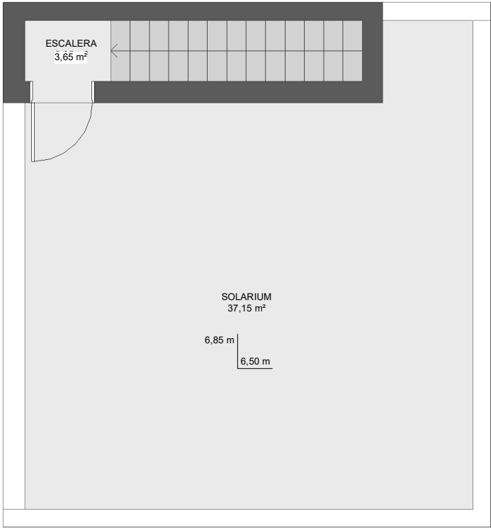
Planta solarium
